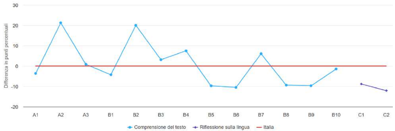
Risposte item per item - Italiano
