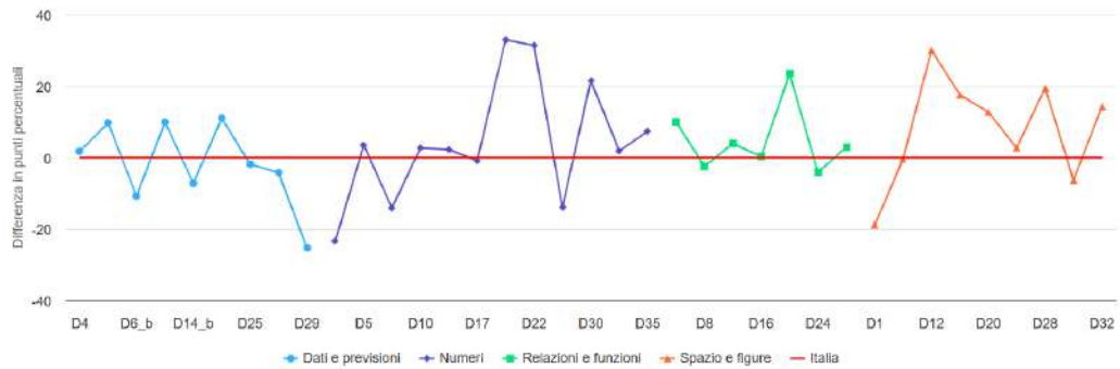
Risposte item per item - Matematica
