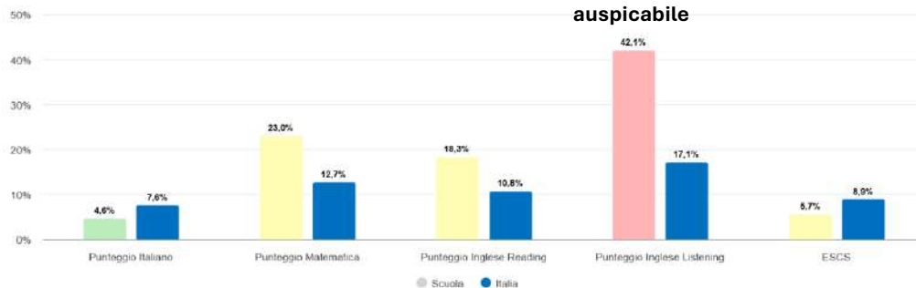
Variabilità tra le classi
